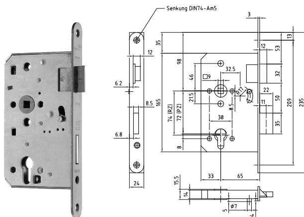
DIN links gezeichnet DIN rechts spiegelbildlich
