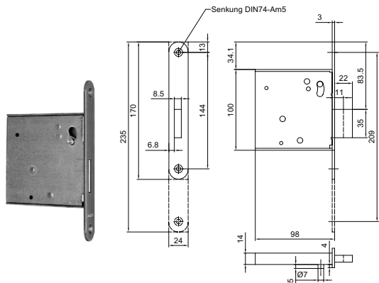
DIN links gezeichnet DIN rechts spiegelbildlich
